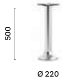
COLUMN Ø 76 TOP MAX 700x700; Ø 900
