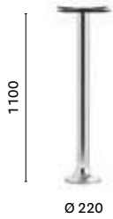
COLUMN Ø 76 TOP MAX 600x600; Ø 700
