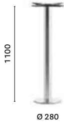
COLUMN Ø 76 TOP MAX 700x700; Ø 900
